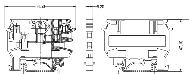
JXB-2-4/35K
