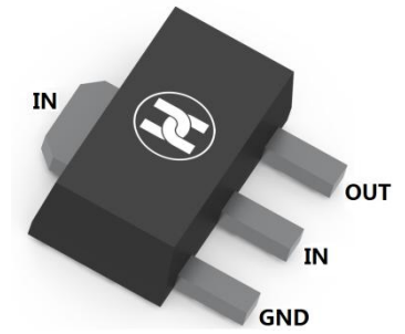
SOT-89
