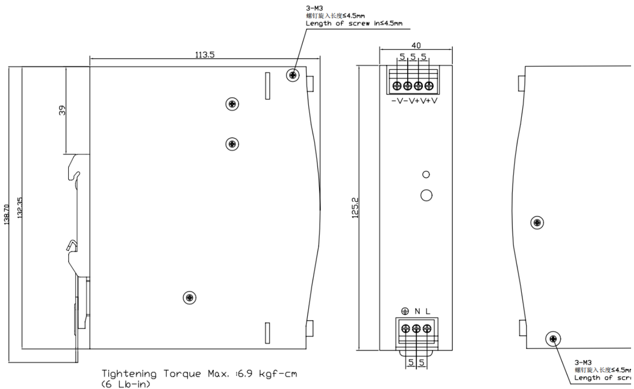
导轨电源SDP1-1AC24-120结构图
