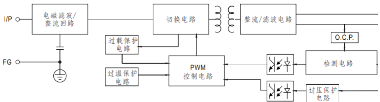
导轨电源SDP1-1AC24-120电气图
