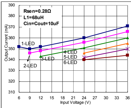
I_{OUT}=350mA Fig. 27
