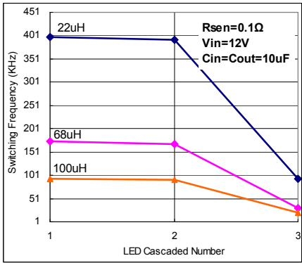
I_{OUT}=1A Fig. 58
