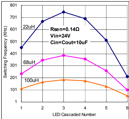
I_{OUT}=1A Fig. 61
