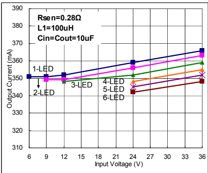
I_{OUT}=350mA Fig. 30
