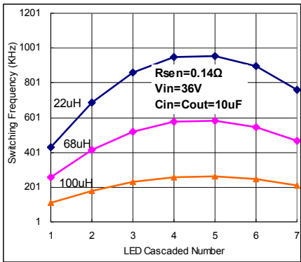
I_{OUT}=1A Fig. 64
