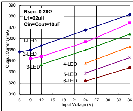
I_{OUT}=350mA Fig. 24
