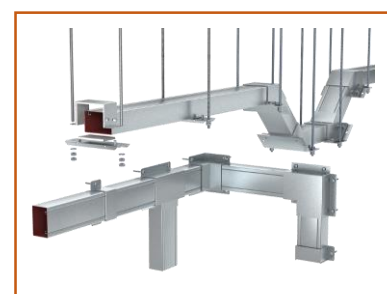
Короб с огнестойким покрытием
