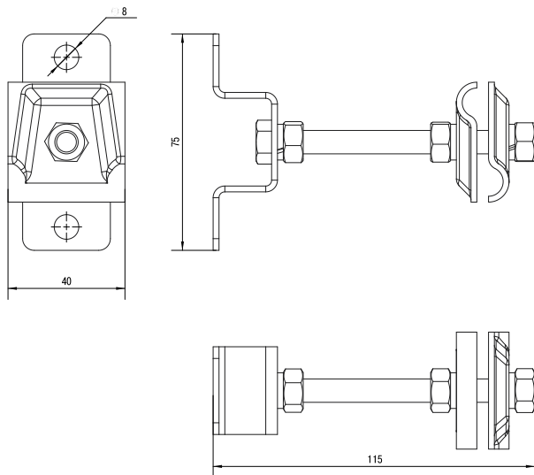
Рисунок 1 – Габаритные размеры
