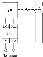
Рисунок 2 – Электрическая схема устройства
