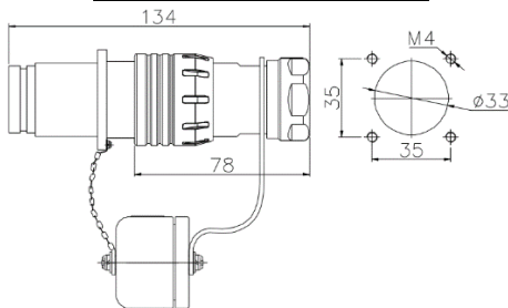
LT-PS-S(NET)/E с креплением на корпус
