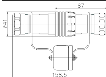
LT-PS-S-x/C с количеством контактов 10, 12, 14, 16, 19 типа «коннектор» (переносной)
