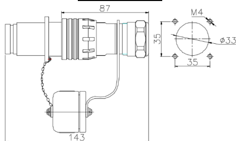
LT-PS-S-x/E с количеством контактов 10, 12, 14, 16, 19 с креплением на корпус
