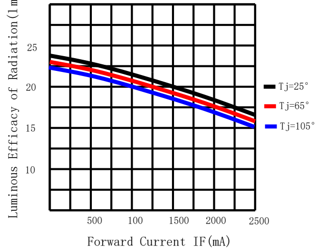
电流-光效曲线
