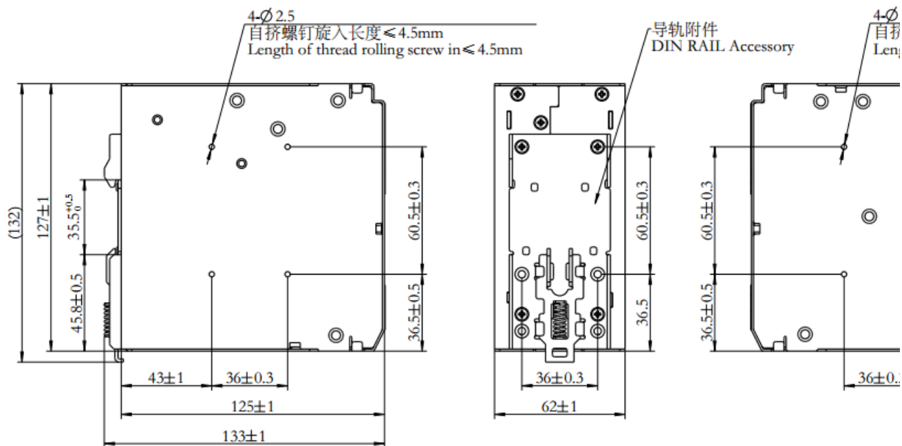
导轨电源SDP2-1AC24-480结构图
