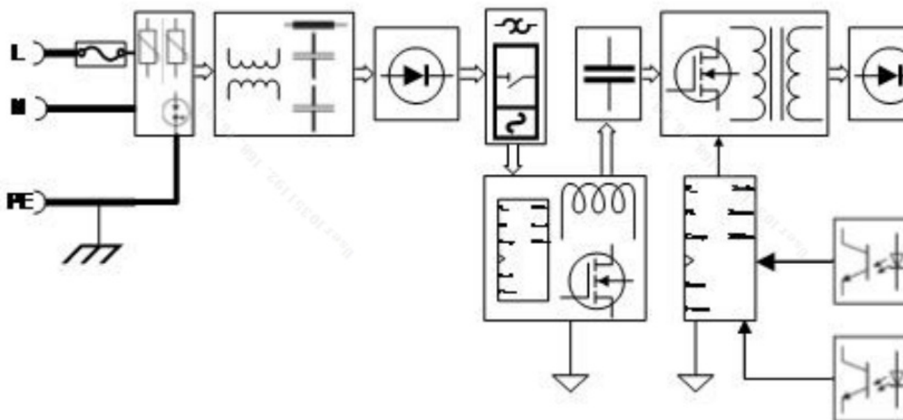
导轨电源SDP2-1AC24-480电气图
