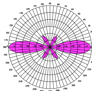
垂直方向图
