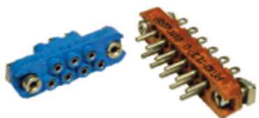
РП10-7 (11,15,22,30,42) З вилка или розетка
