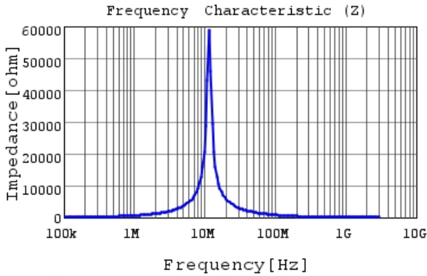
LQH3NPZ101MME |Z|
