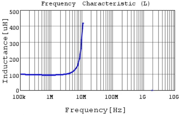
LQH3NPZ101MME L
