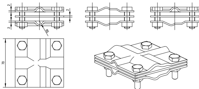
Рисунок 1 – Габаритные размеры
