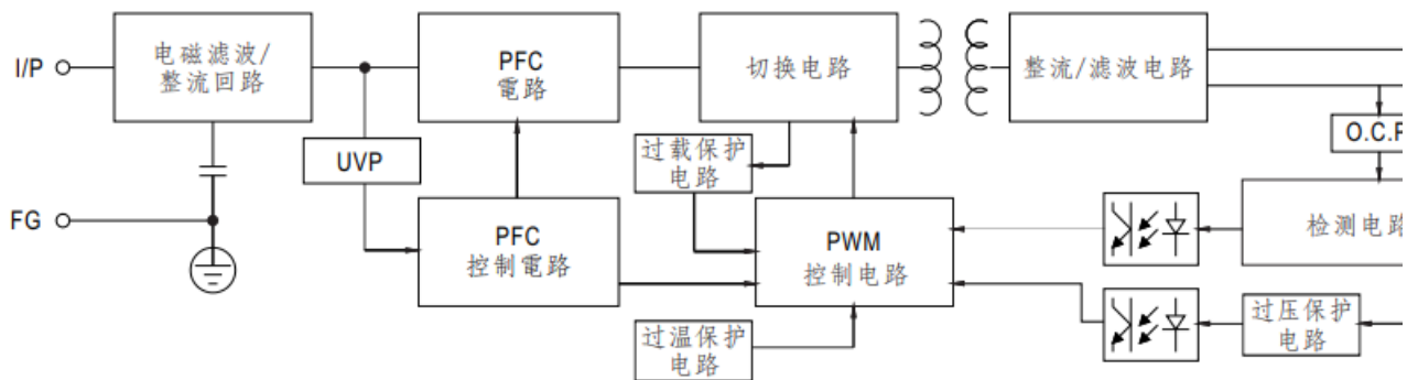
导轨电源SDP1-1AC24-480电气图
