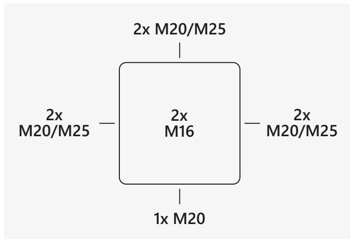
Схема расположения выбивных отверстий
