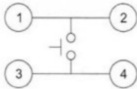
Схема коммутации
