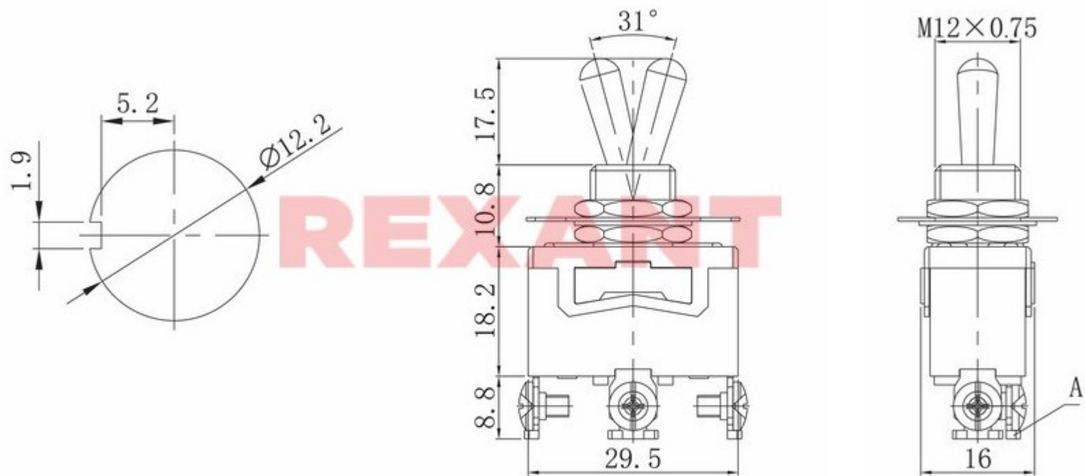
Тумблер 250V 15A (3c) ON-OFF-ON однополюсный REXANT
