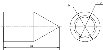
Рисунок 1 – Габаритные размеры
