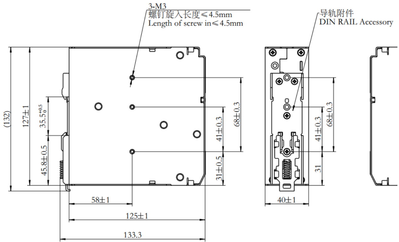
导轨电源SDP2-1AC24-240结构图
