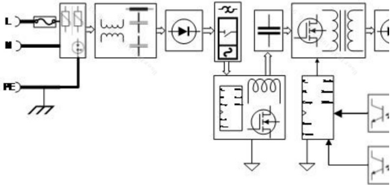
导轨电源SDP2-1AC24-240电气图
