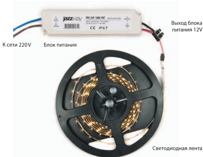
СХЕМА 1. Как подключить светодиодную ленту
