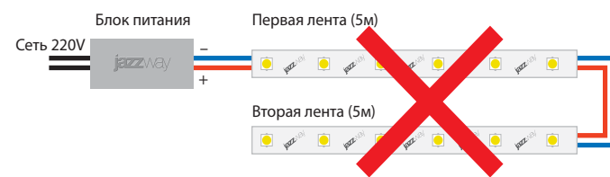
СХЕМА 2. Так подключать нельзя!
