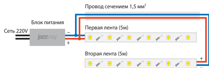
СХЕМА 3. Правильное подключение нескольких светодиодных лент к одному блоку питания
