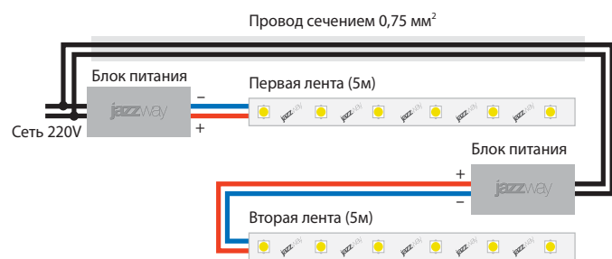
СХЕМА 4. Подключение светодиодной ленты с двумя блоками питания
