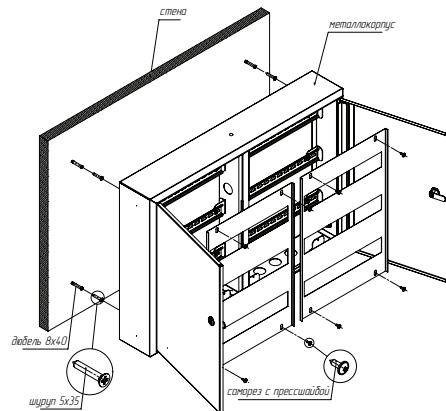
Рис. 1 - Схема монтажа
