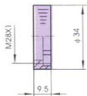
WIRE(L) TYPE
