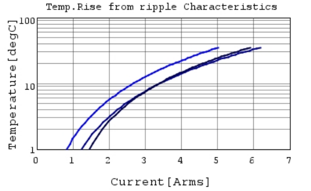
GRM32EC72A106KE05 Temp.rise — 80kHz —
