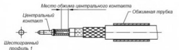
Схема кримпирования разъемов типа BNC/ TNC на коаксиальный кабель
