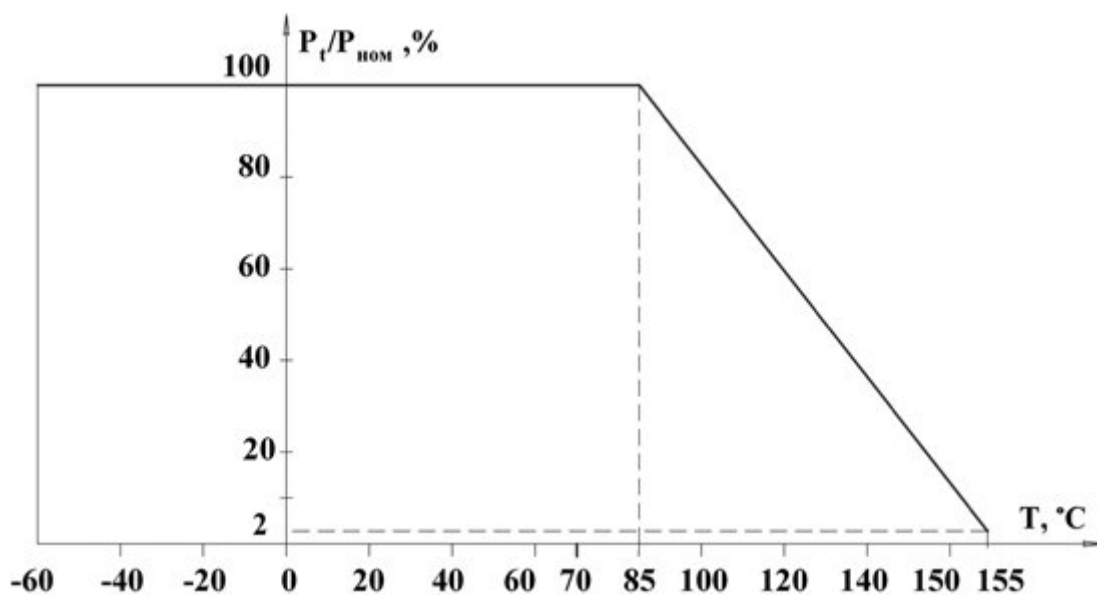
Рис. 1. При наработке: до 1000 ч. для C2-29В-0.5М; C2-29В-1-Н; C2-29В-2-Н (с допуском отклонением \pm 0,5; \pm 1\% ); до 10 000 ч. для C2-29В-0.062; до 25 000 для C2-29В-0.125, C2-29В-0.25.
