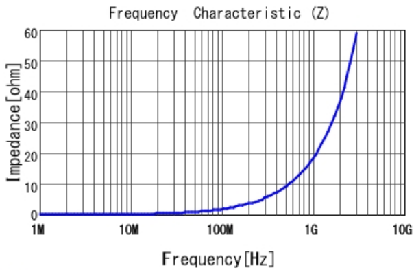
■ LQW15AN3N0C80 |Z|
