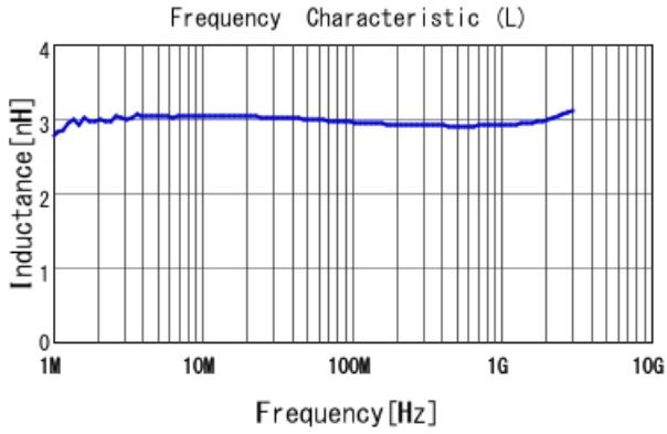
■ LQW15AN3N0C80 L
