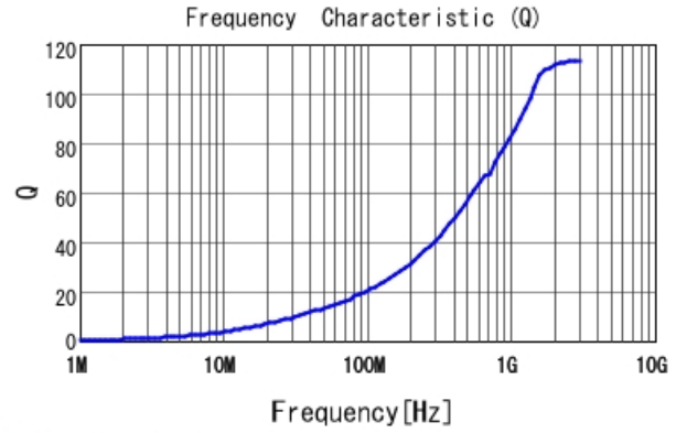
■ LQW15AN3N0C80 Q
