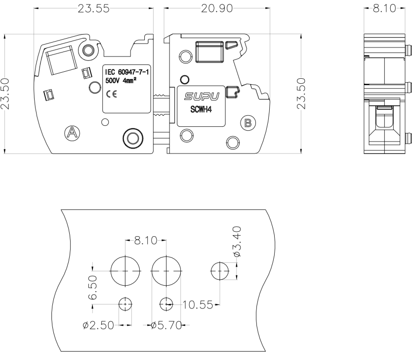
钻孔图
