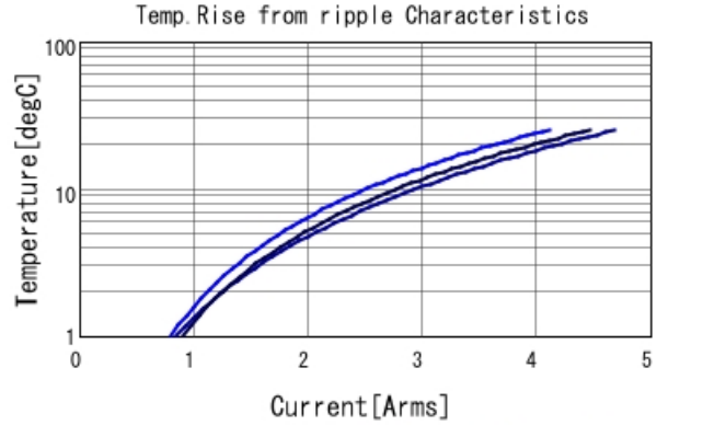
KRM55QR72A106KH01 Temp. rise ■ 50kHz ■ 100kHz ■ 300kHz
