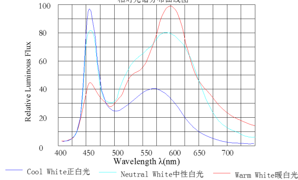
Wavelength Characteristics Ta=115°C 相对光谱分布曲线图
