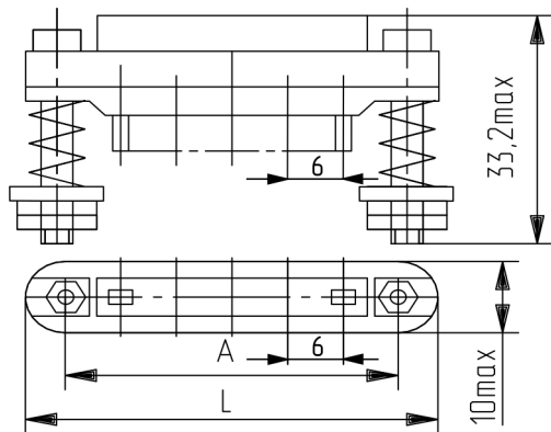
Рисунок 2 Розетка однорядная
