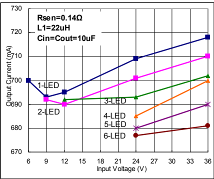
I_{OUT}=700mA Fig. 23
