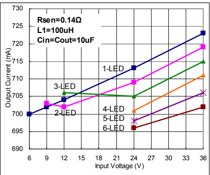
I_{OUT}=700mA Fig. 29
