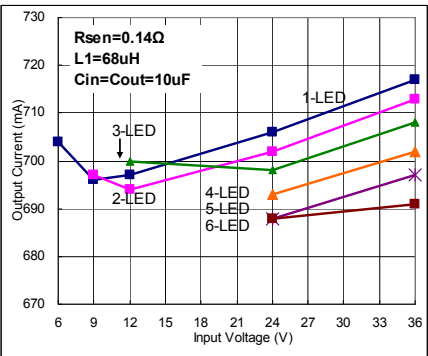
I_{OUT}=700mA Fig. 26
