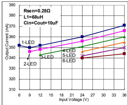
I_{OUT}=350mA Fig. 27
