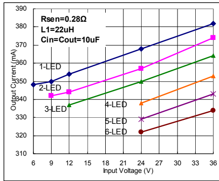
I_{OUT}=350mA Fig. 24
