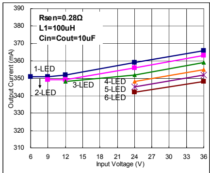
I_{OUT}=350mA Fig. 30
