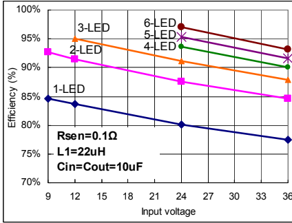
I_{OUT}=1A
