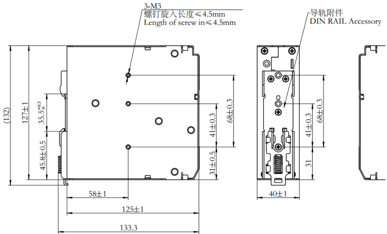
导轨电源SDP1-1AC24-240结构图
