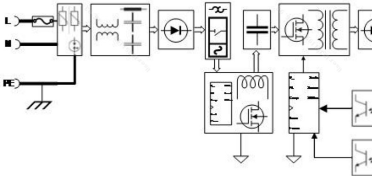
导轨电源SDP1-1AC24-240电气图
