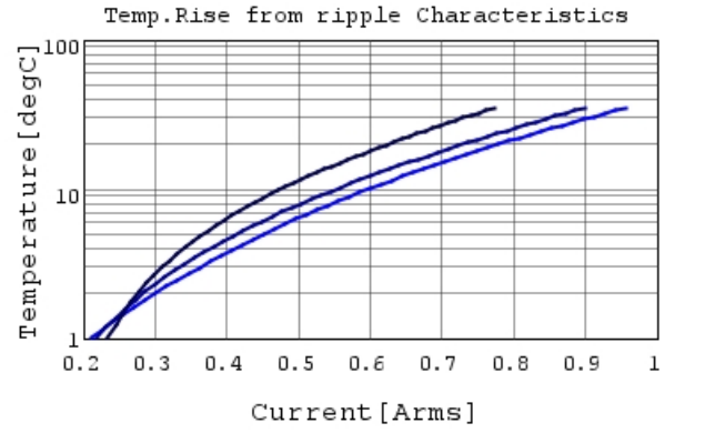
GRM1555C1H8R0BA01 Temp.rise 700MHz
