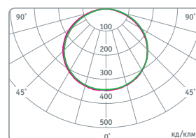
NHB-P5-200-5K-120D-LED
