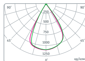
NHB-P5-150-5K-60D-LED
