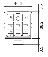
062.07 с реле
