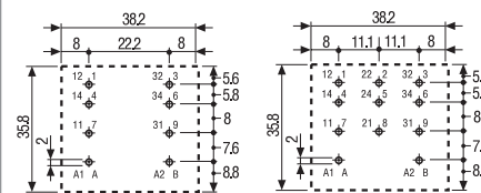
62.22 Вид сбоку
