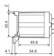
062.07 с реле
