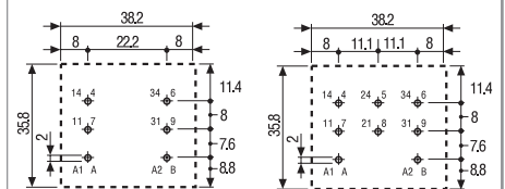
62.22 - 0300 Вид сбоку
