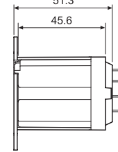
062.05 с реле
