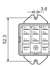
062.05 с реле
