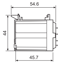
062.08 с реле
