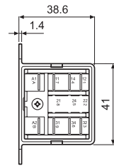
062.60 с реле
