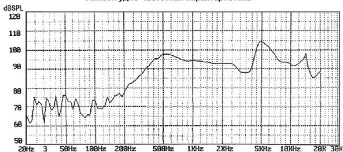
Амплитудно-частотная характеристика
