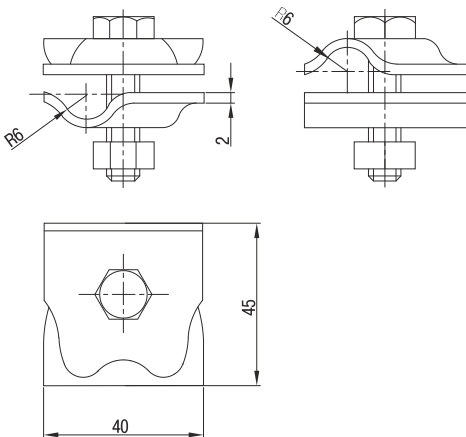
Рисунок 1 – Габаритные размеры
