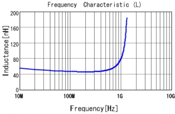
■ LQG15HS47NJ02 L
