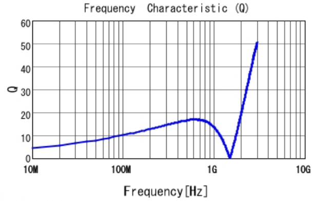
■ LQG15HS47NJ02 Q
