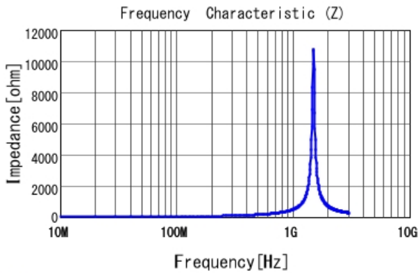
■ LQG15HS47NJ02 |Z|
