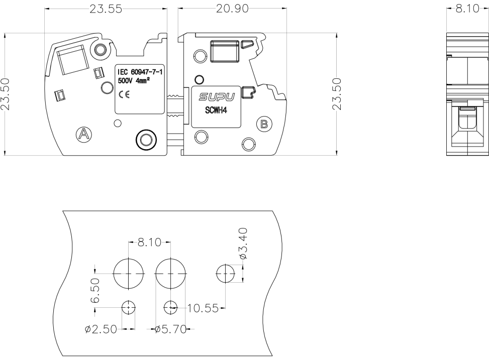
钻孔图
