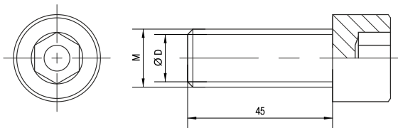
Рисунок 1 – Габаритные размеры
