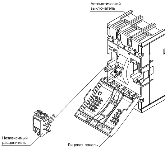
Рисунок 3 – Установка устройств в выключатели ВА88 серии MASTER на примере РНм-250
