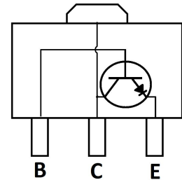
SOT-89
