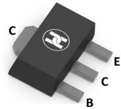
SOT-89
