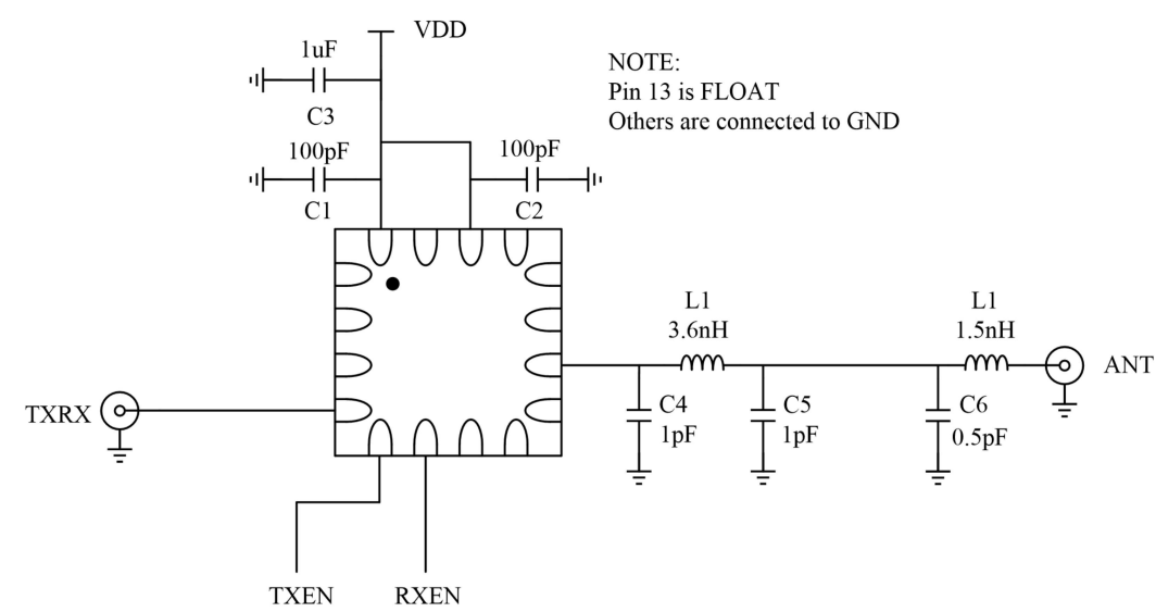
图 4-4 芯片应用电路图 2
